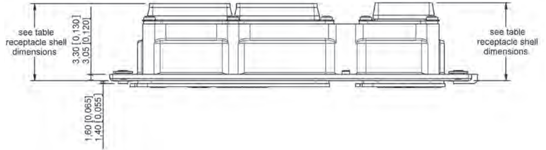
RECEPTACLE SHELL
